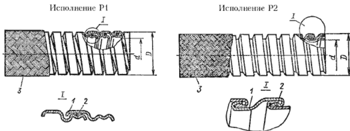
Рис.2.2. Металлические рукава: 1 - профилированная лента; 2 - уплотнитель; 3 - проволочная оплетка
