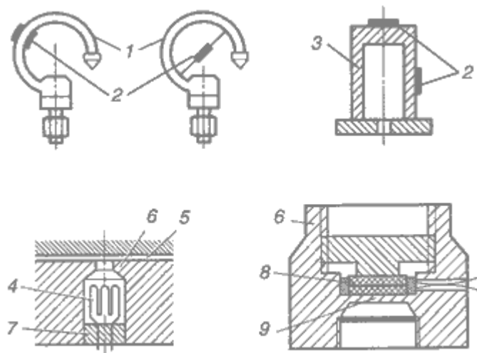
Рис.7.34. Электрические манометры:
