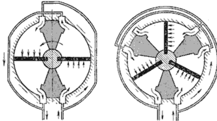
Рис.4.8. Поворотные гидроцилиндры: а - двухлопастной; б - трехлопастной
