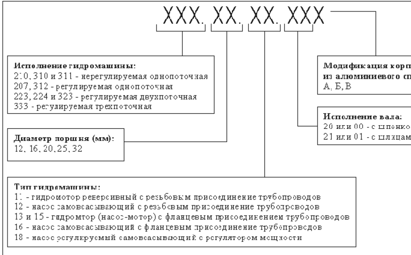
Рис.3.11. Структура условного обозначения аксиально-поршневых гидромашин серий 200 и 300
