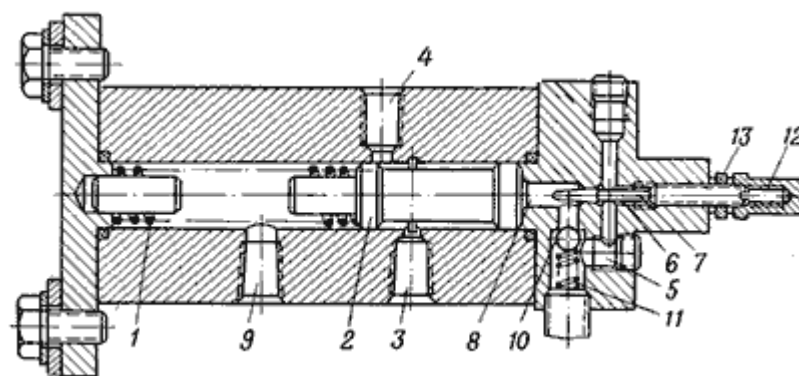
Рис.7.28. Реле времени дроссельного типа 1, 11 - пружины; 2 - золотник; 3, 4 - подводящее и отводящее отверстия; 5, 8 - полости; 6 - канал; 7 - дроссель; 9 - сливное отверстие; 10 - шарик; 12 - колпачок; 13 - контрогайка
