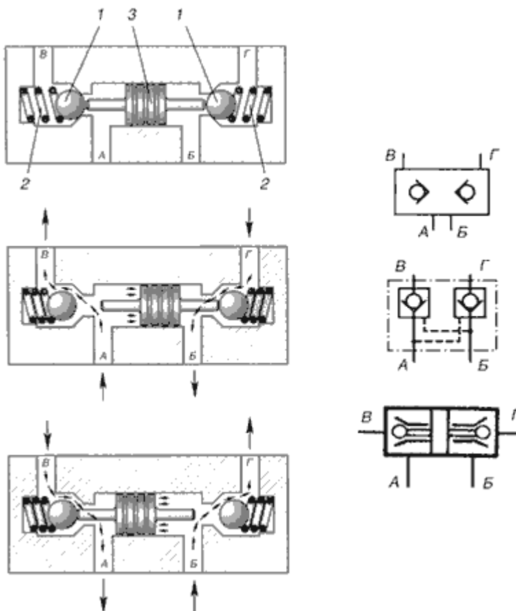
Рис.7.24. Двухсторонний гидрозамок: а - нейтральное положение; б - положение толкателя при подводе давления в канал А; в - положение толкателя при подводе давления в канал В; г - условные обозначения
