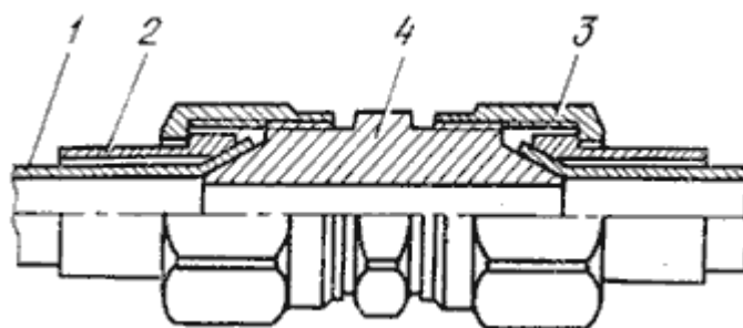
Рис.2.3. Соединение по наружному конусу
