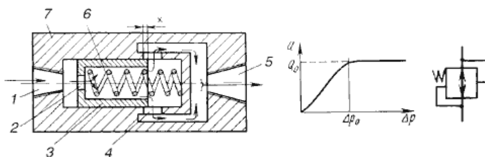
Рис.6.8. Ограничитель расхода: а - принципиальная схема; б - зависимость Q=f(\Delta P) ; в - условное обозначение
