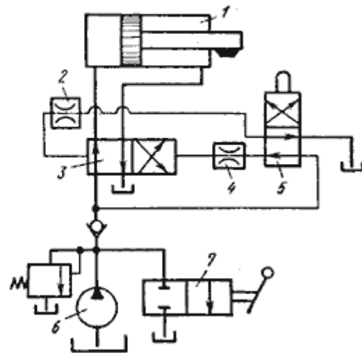
Рис.10.5. Гидросистема с двухступенчатым (пилотным) распределением и ручной разгрузкой
