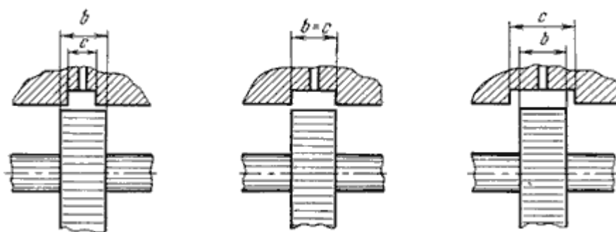
Рис.5.7. Конструктивные исполнения золотников
