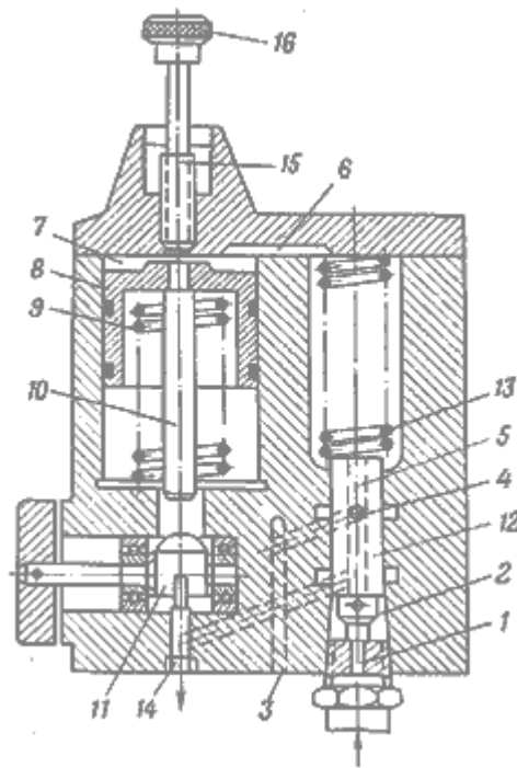
Рис.7.29. Реле времени объемного типа 1, 4 - отверстия; 2, 6, 7 - полости; 3, 5 - каналы; 8 - поршень; 9, 13 - пружины; 10 - шток; 11 - упор; 12 - золотник; 14 - сливное отверстие; 15 - винт; 16 - рукоятка
