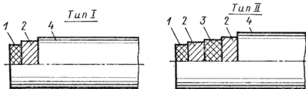
Рис.2.1. Схемы конструкции рукавов с оплеткой: 1 - внутренний резиновый слой; 2 - металлическая оплетка; 3 - промежуточный резиновый слой; 4 - наружный резиновый слой
