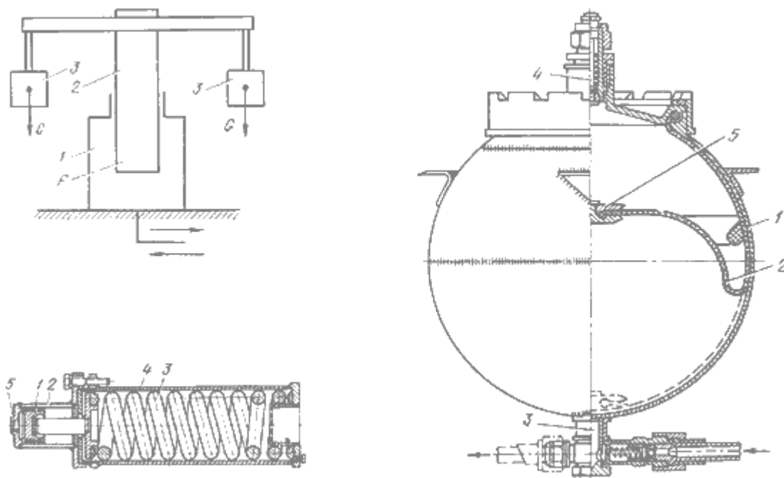
Рис.7.21. Гидроаккумуляторы:
