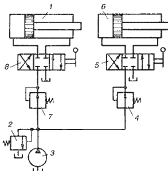
Рис.10.12. Гидросистема с двумя гидроцилиндрами, питаемыми одним насосом через редуцирующие клапаны
