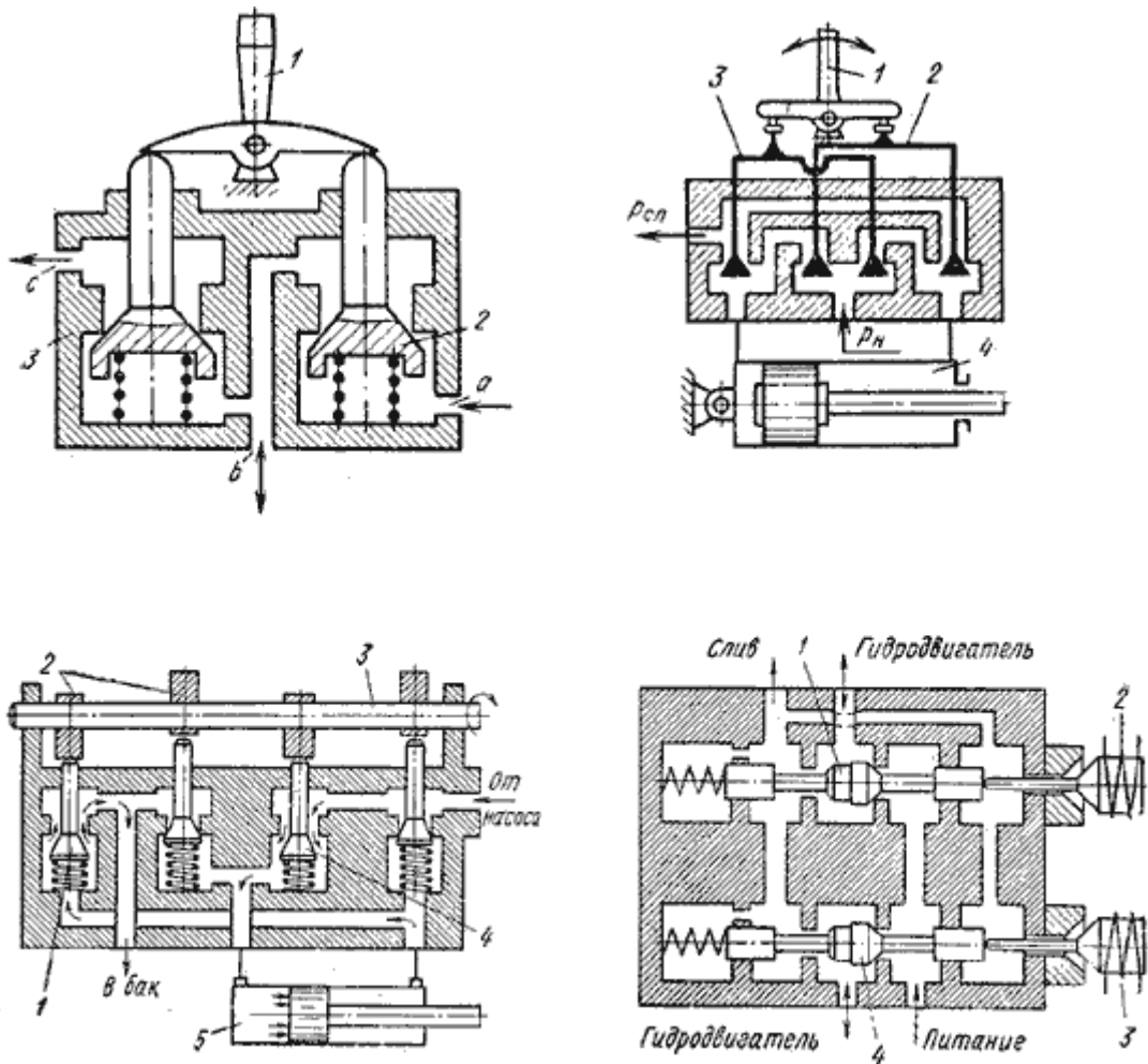
Рис.5.10. Клапанные распределители: а, б - с качающимся рычагом; в - с кулачковым приводом; г - с электромагнитным приводом
