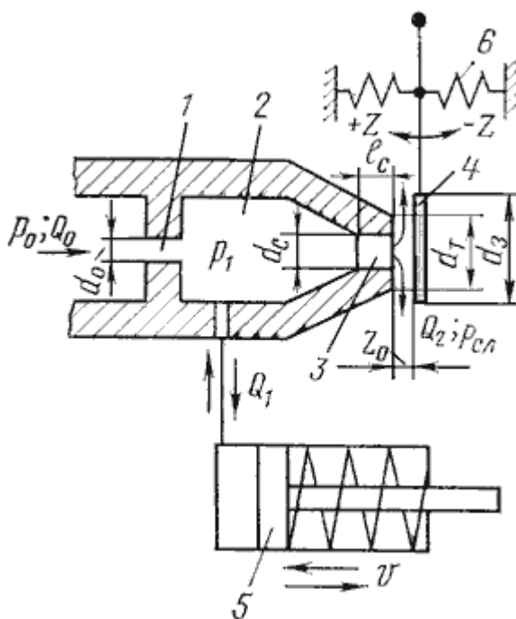
Рис.8.4. Гидроусилитель с соплом и заслонкой:
