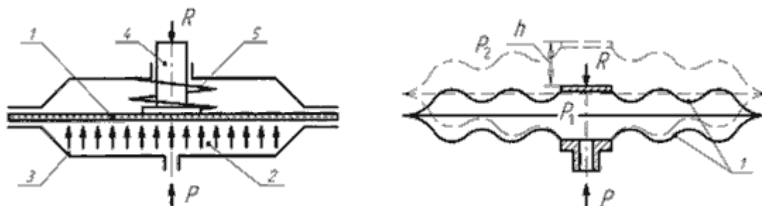
Рис.4.1. Схемы мембран:
