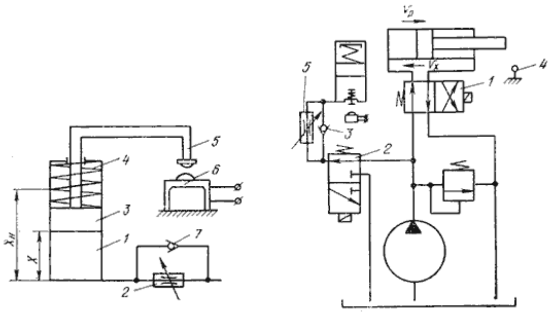
Рис.7.27. Реле времени: а - принципиальная схема; б - вариант схемы включения
