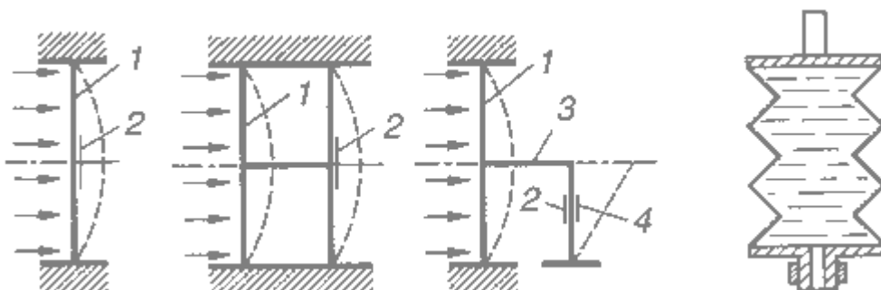
Рис.7.32. Деформационные манометры: а - мембранный; б - мембранный с двойной мембраной; в - с консольной балкой; г - сильфонный; 1 - мембрана; 2, 4 - активный и компенсирующий тензорезистор; 3 - консольная балочка
