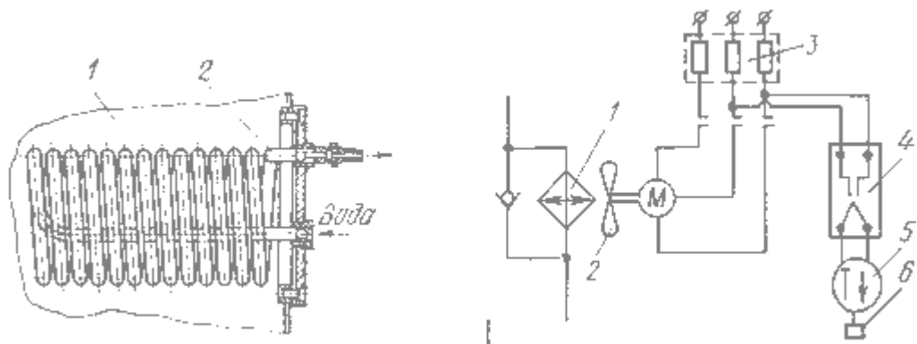
Рис.7.2. Теплообменники:
