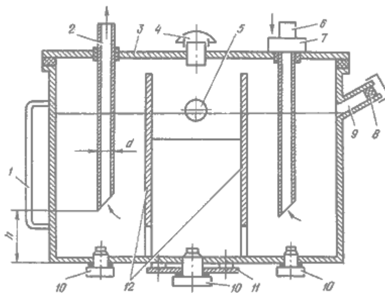
Рис.7.1. Гидробак:
