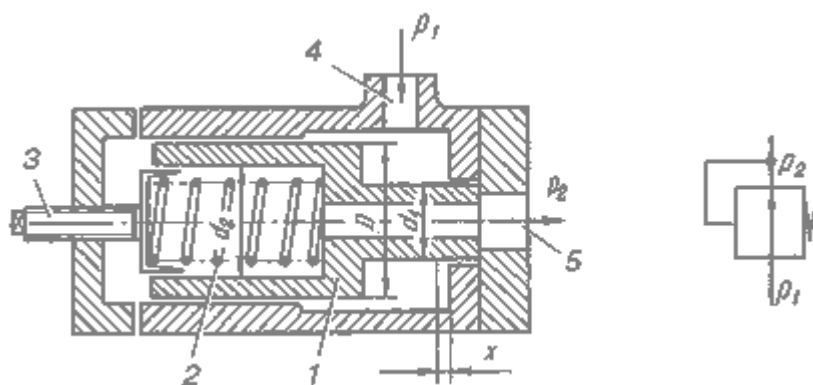
Рис.6.4. Редукционный клапан: а - принципиальная схема; б - условное обозначение
